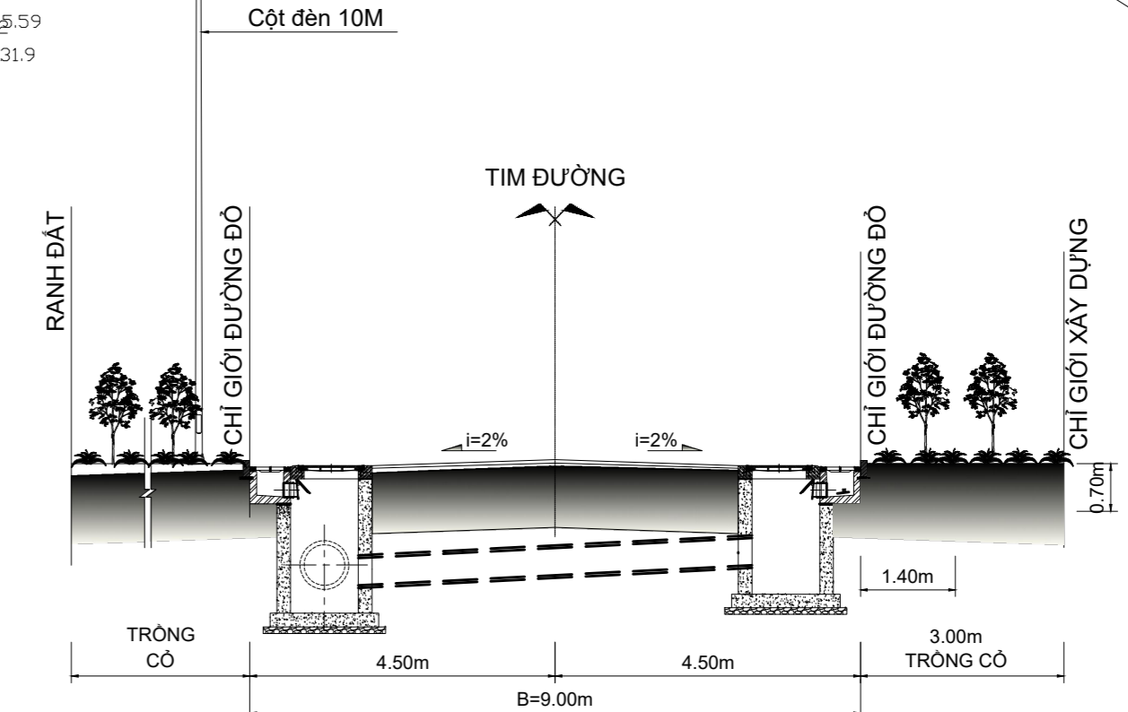
MẶT CÁT 1-1 (VỊ TRÍ CỘT HỒ THU NƯỚC)
