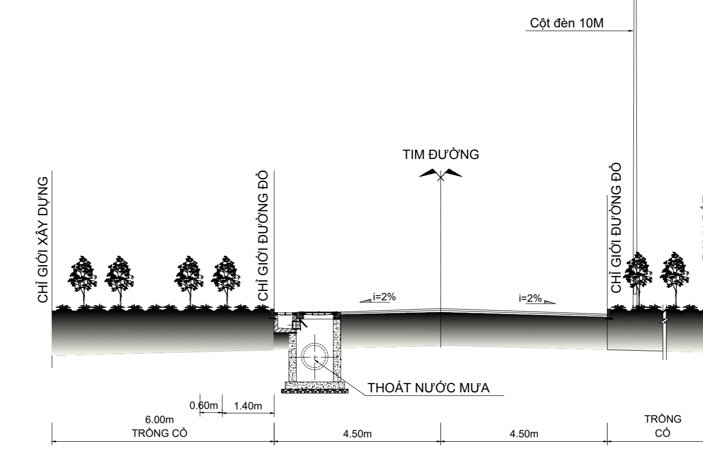
MẶT CÁT 2-2 (VỊ TRÍ CỘT HỒ THU NƯỚC)
