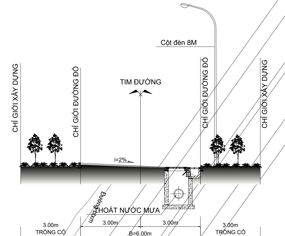
MẶT CÁT 3-3 (VỊ TRÍ CỘT HỒ THU NƯỚC)
