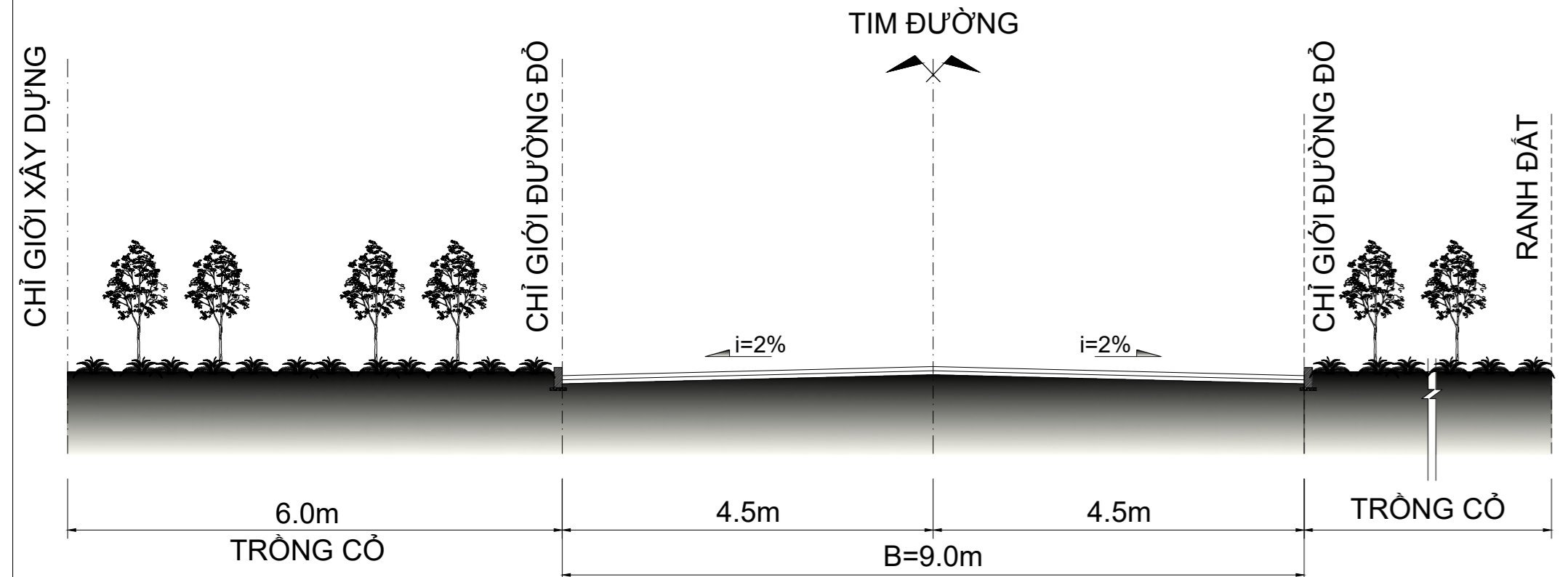
MẶT CẮT 2-2
