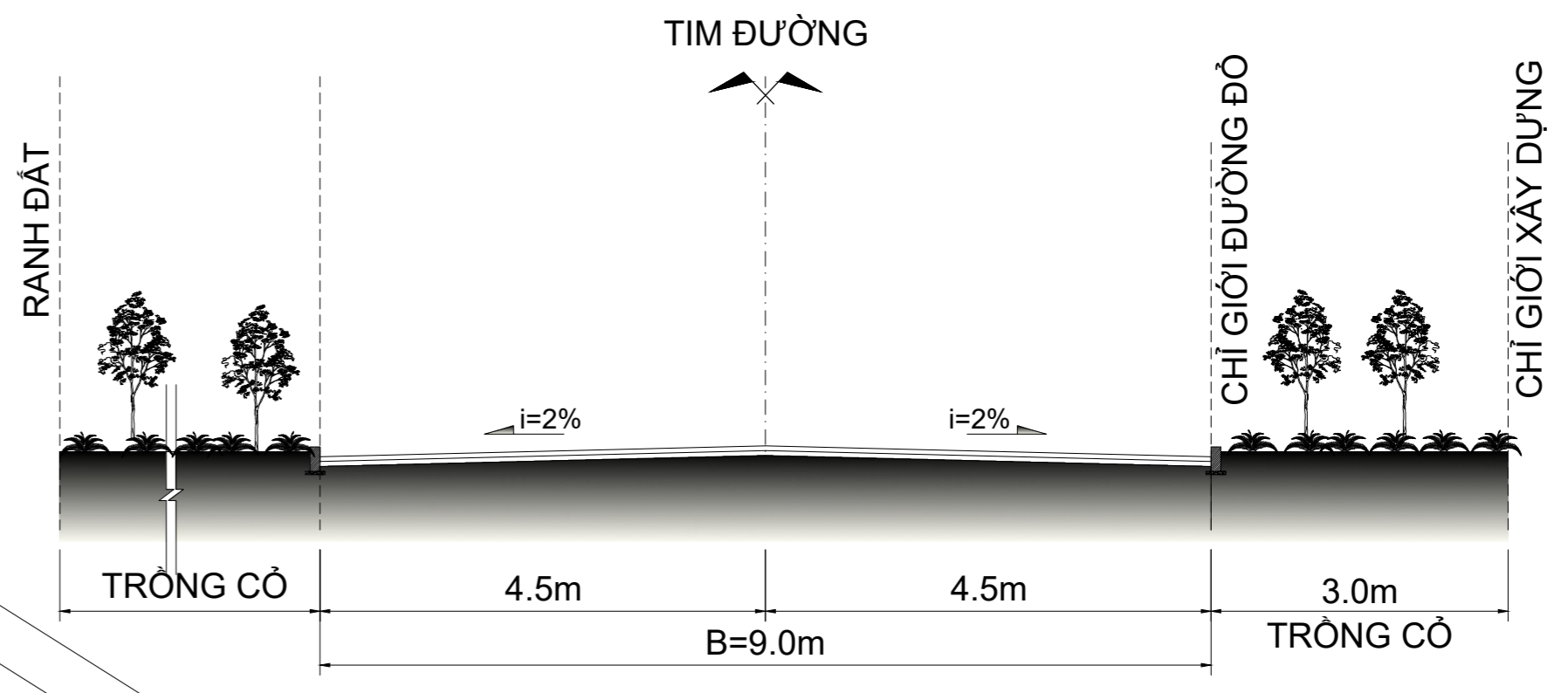
MẶT CẮT 1-1
