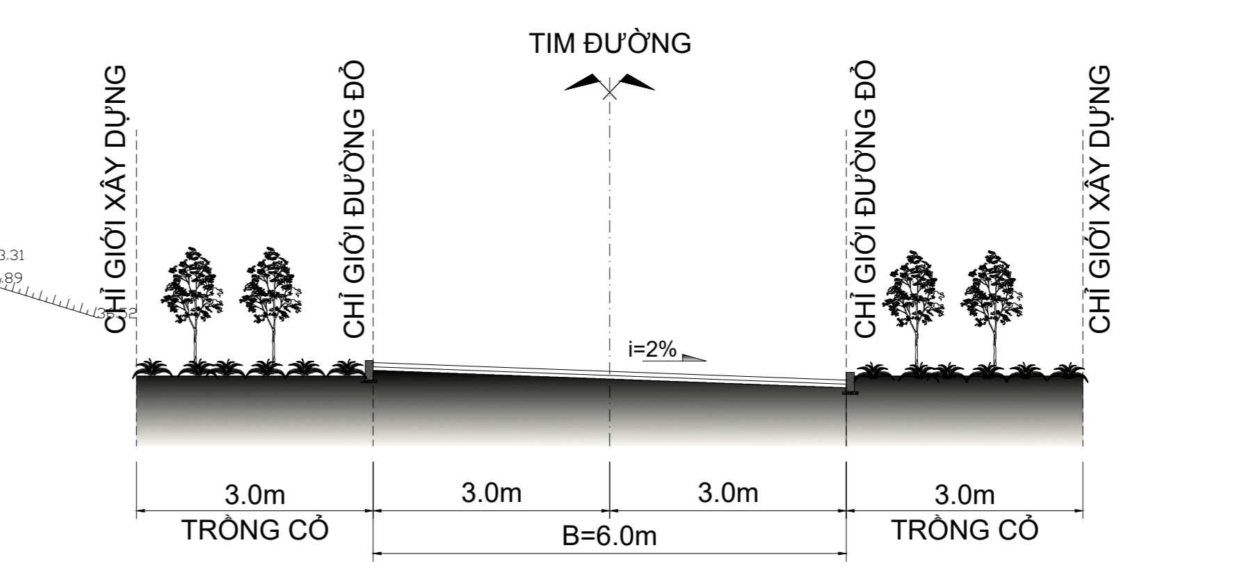
MẶT CẮT 3-3
