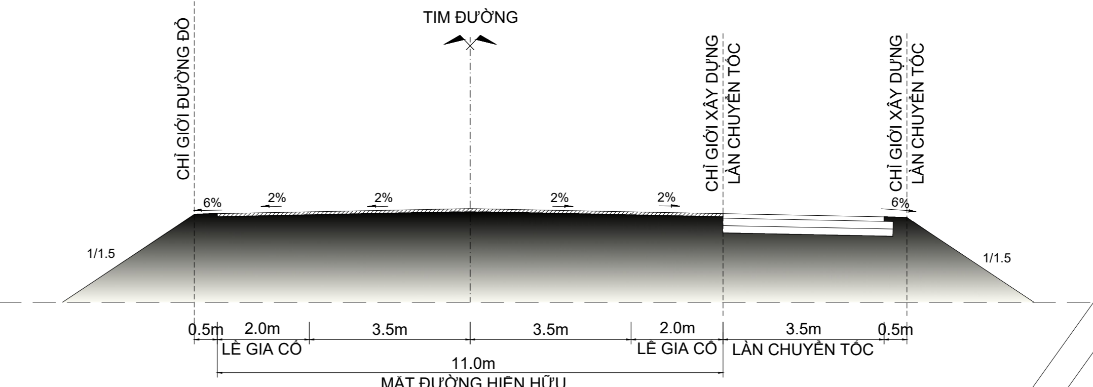
MẶT CẮT 4-4 (LÀN CHUYẾN TỐC TRÊN TUYẾN TRÁNH QL19)
