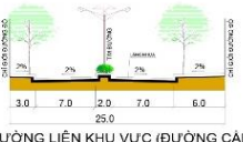
6C-6C ĐƯỜNG LIÊN KHU VỰC (ĐƯỜNG CÁN VƯƠNG) LỘ GIỚI TỪ 22 - 25M (TÙY ĐOẠN)
