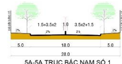
5A-5A TRỤC BẮC NAM SỐ 1 (ĐOẠN TỪ ĐT.638 ĐẾN CẦU MỜI) ĐT.638 (TỪ QL.19 QUA NHƠN LỘC ĐẾN NHƠN PHÚC)
