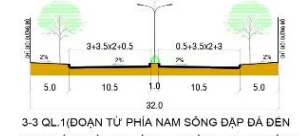
3-3 QL.1 (ĐOẠN TỪ PHÍA NAM SÔNG ĐÁP ĐÁ ĐẾN GIAO VỚI ĐƯỜNG TRÁNH) - ĐƯỜNG TRỤC CHÍNH ĐÔNG TÂY SỐ 2
