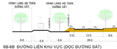
6B-6B ĐƯỜNG LIÊN KHU VỰC (ĐỌC ĐƯỜNG SẮT)
