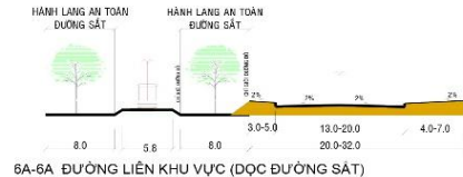
6A-6A ĐƯỜNG LIÊN KHU VỰC (ĐỌC ĐƯỜNG SẮT)
