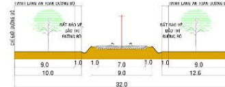
IV-IV ĐƯỜNG CẤP IV
