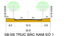
5B-5B TRỤC BẮC NAM SỐ 1 (ĐOẠN TỪ CẦU KHÁNH MỸ ĐẾN QL.19B)
