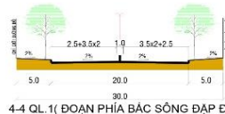
4-4 QL.1 (ĐOẠN PHÍA BẮC SÔNG ĐÁP ĐÁ) QL.19, QL.19B, ĐT.631, ĐT.636
