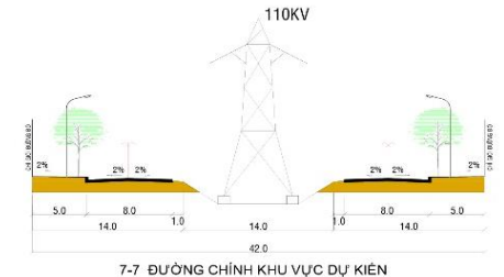
7-7 ĐƯỜNG CHÍNH KHU VỰC DỰ KIẾN
