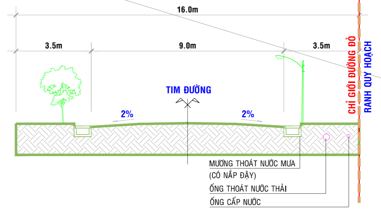
MẶT CẮT 2-2
