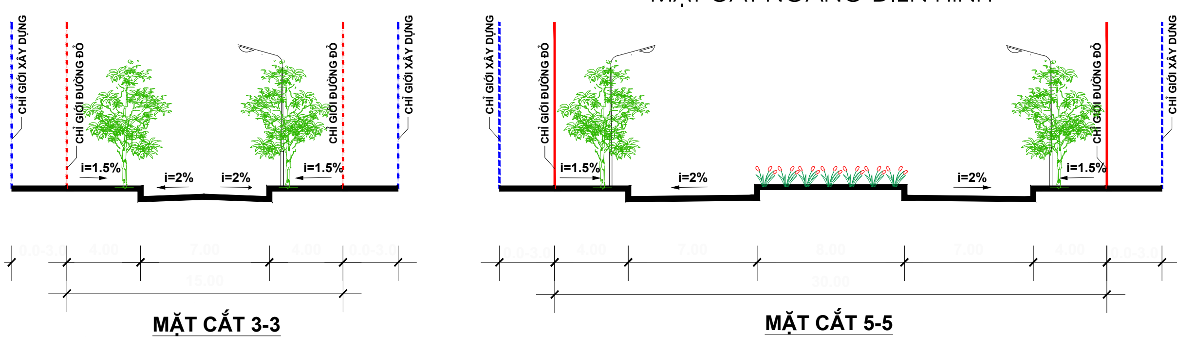
MẶT CẮT NGANG ĐIỂN HÌNH
