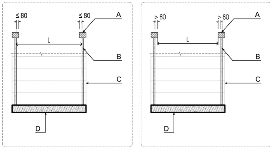
Hình A.26 – Cách xác định chiều rộng tính toán thoát nạn của vé thang (trường hợp trống cả hai bên vé thang)
