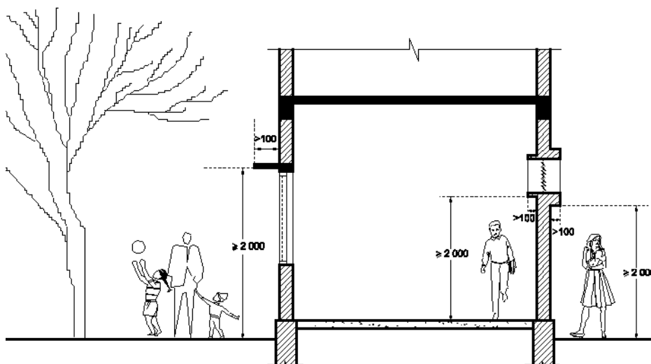
Hình A.10 – Chiều cao thông thủy các bộ phận nhô ra
